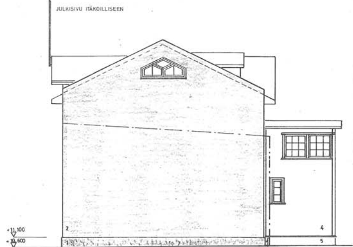
PÄÄTY LÄNSILOUNAASEEN
