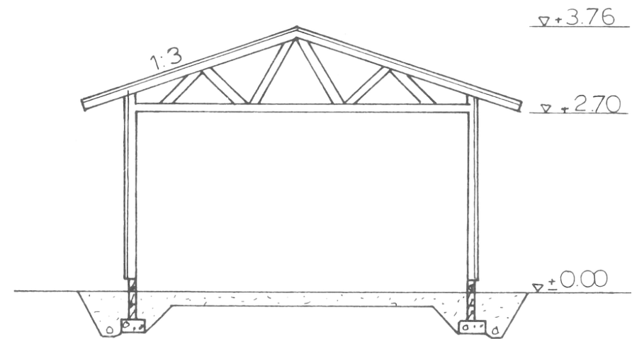
LEIKKAUS A-A
