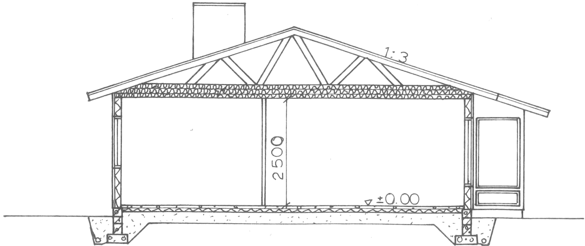
LEIKKAUS A-A
