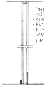
VÄLISEINÄ 1:10
